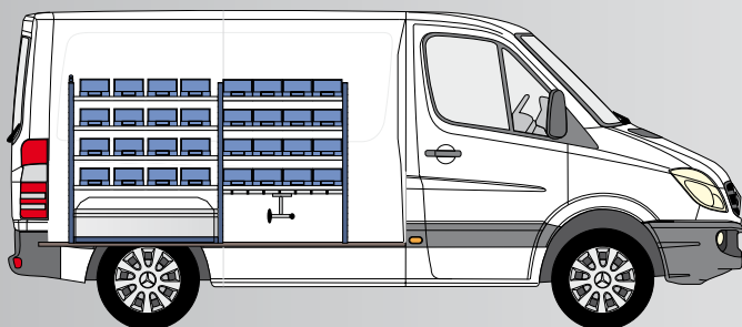
Mercedes Sprinter mit Einbau PL 569, links
